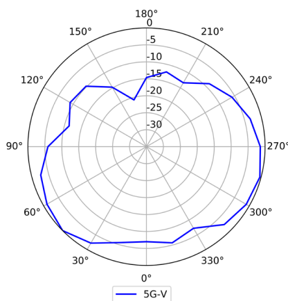
5G (Vertical)
