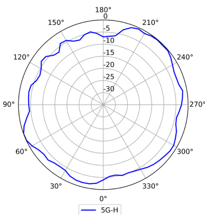
5G (Horizontal)
